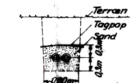
Tværsnit af varmekanal 1:50
