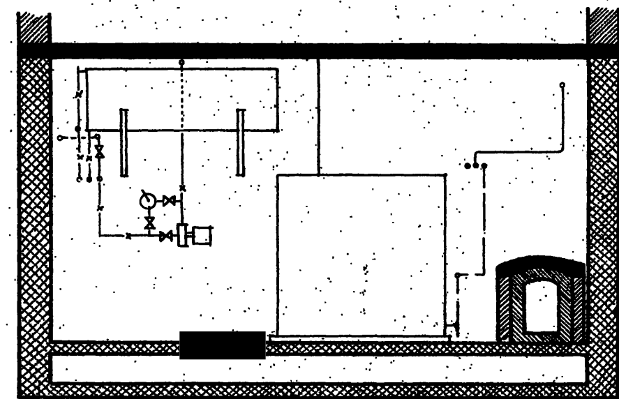
Snit B-B
