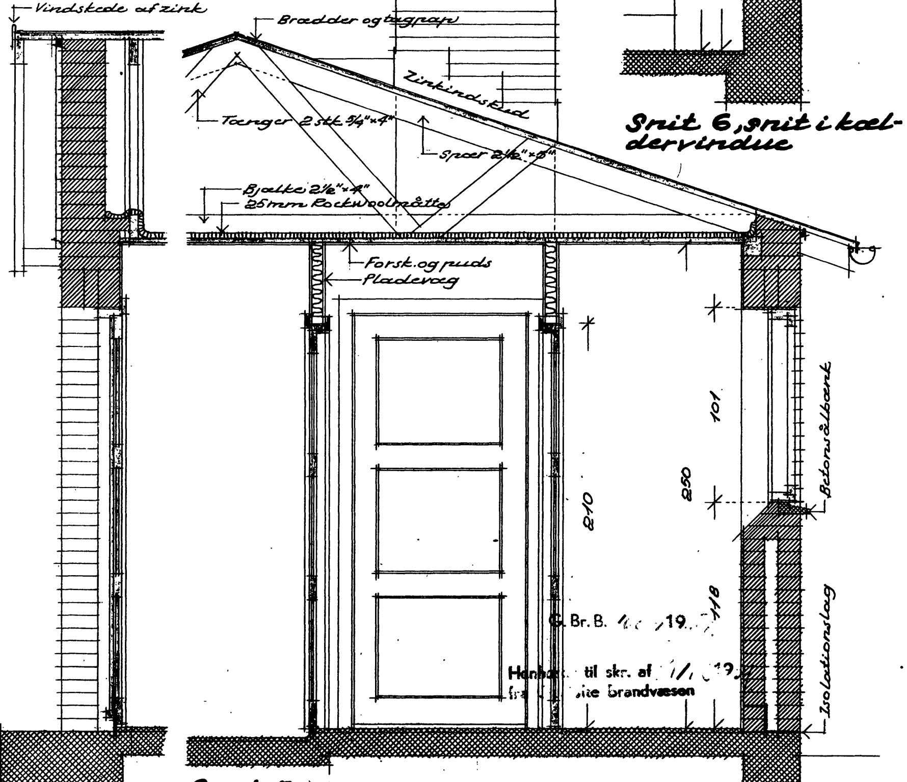
Snit 5, tværsnit.
